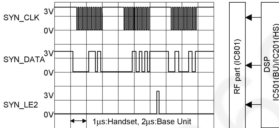
SYN_CLK & SYN_DATA
