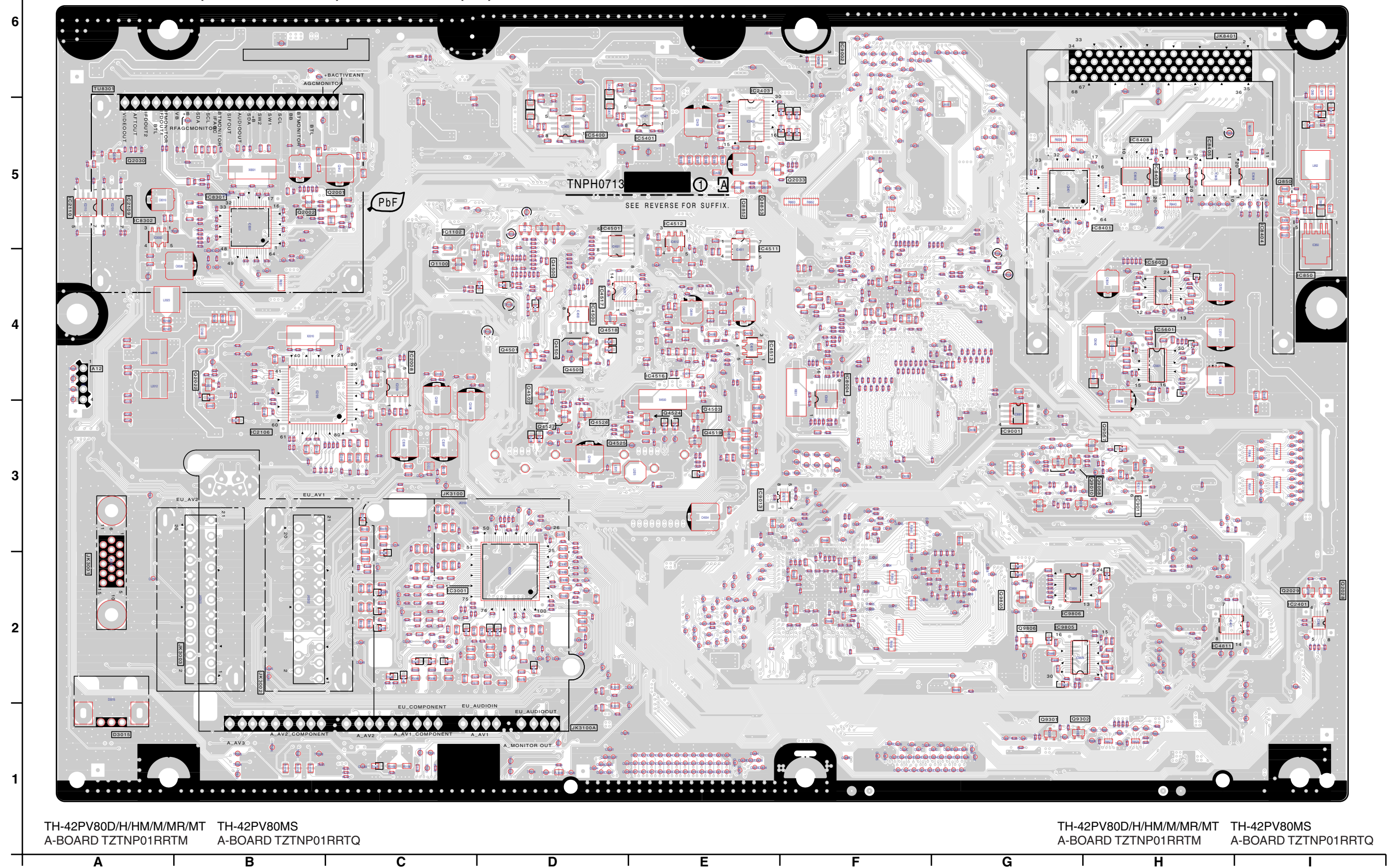
A-BOARD (FOIL SIDE) TZTNP01RRTM(D/H/HM/M/MR/MT) TZTNP01RRTQ(MS)
