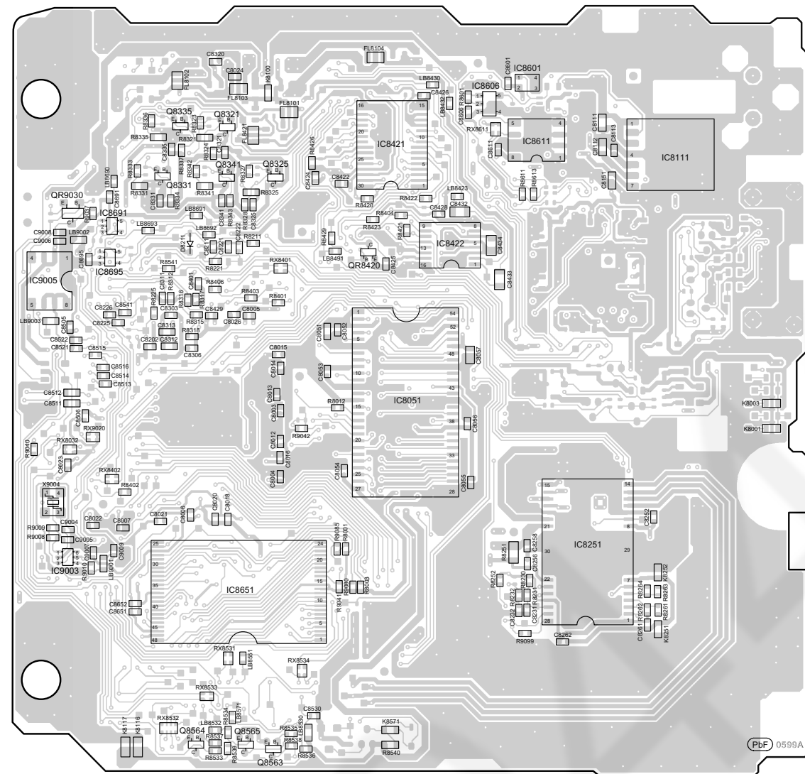
A DVD MODULE P.C.B. (RFKBX0681F-C)
