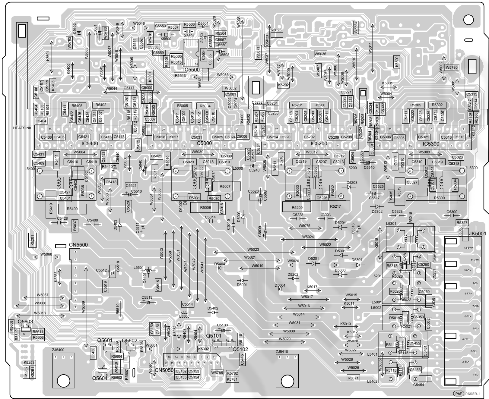
M D-AMP P.C.B. (REPX0731B)
