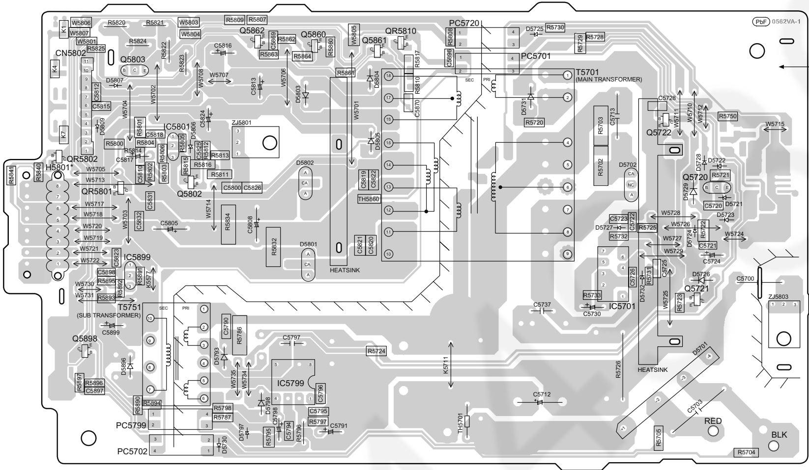
N SMPS P.C.B. (REPX0751E)
