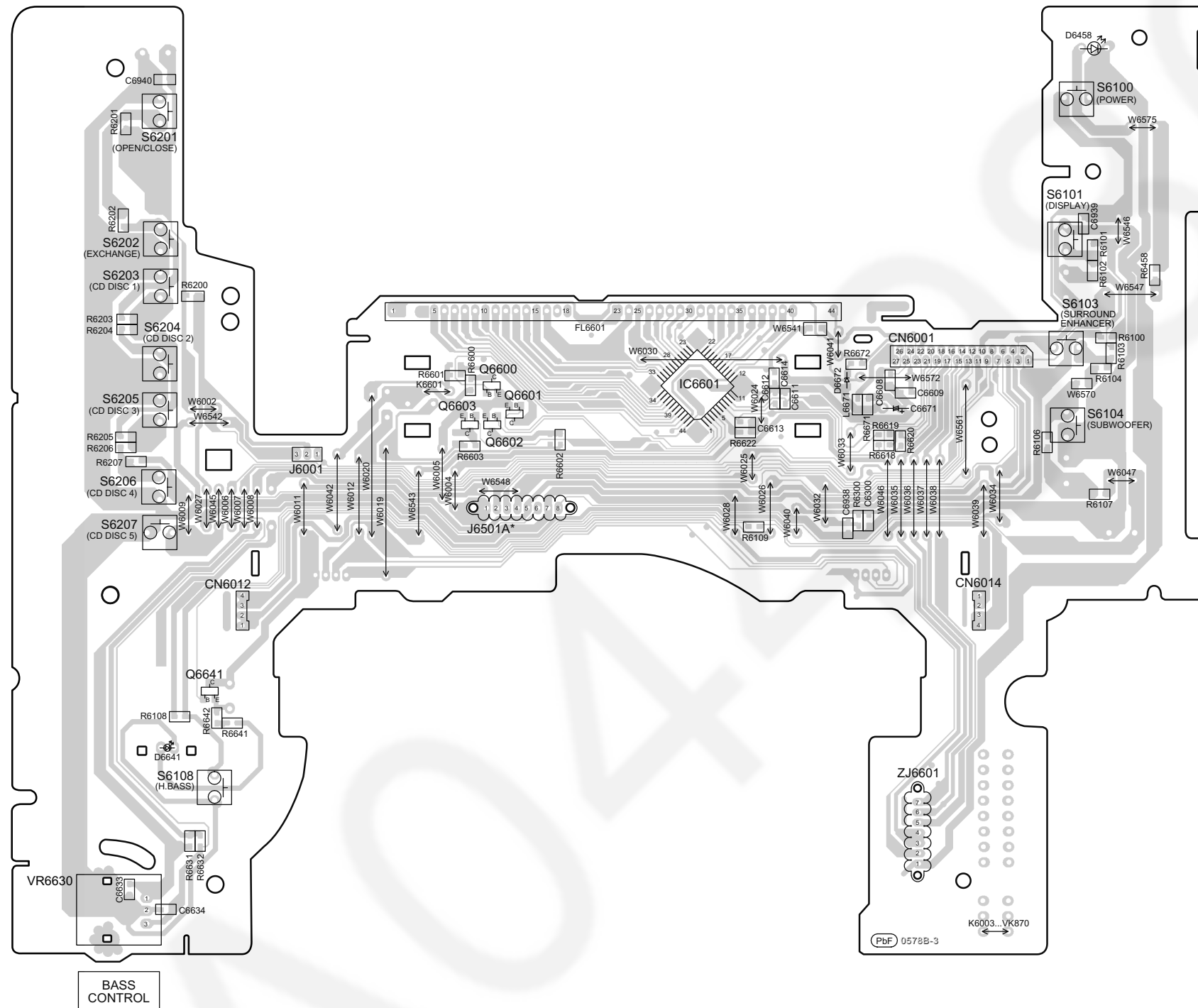
C PANEL P.C.B. (REPX0671C)
