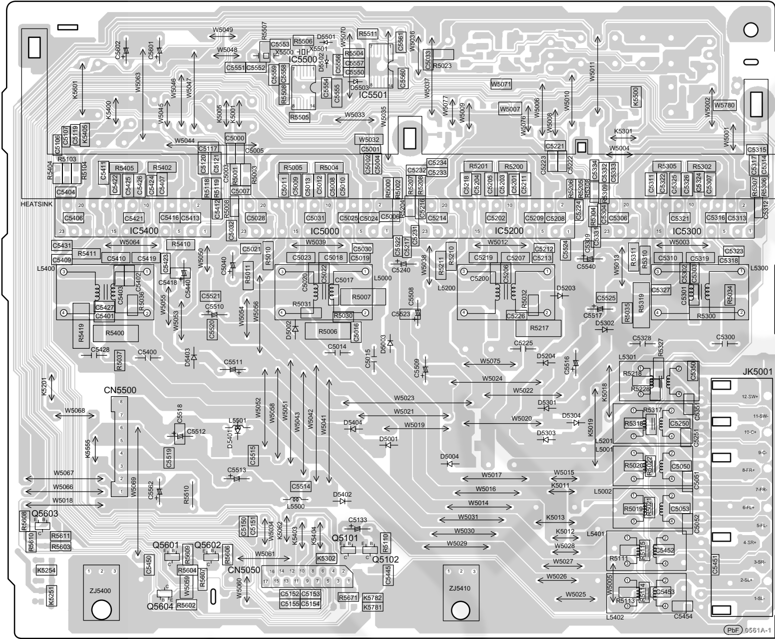
M D-AMP P.C.B. (REPX0638D)
