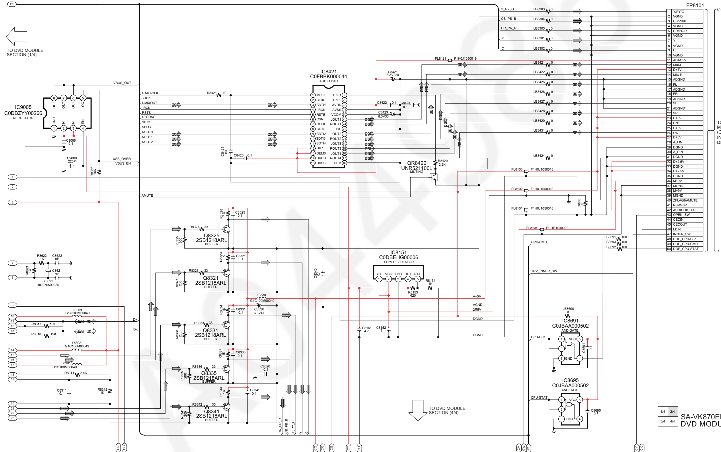
A DVD MODULE CIRCUIT
