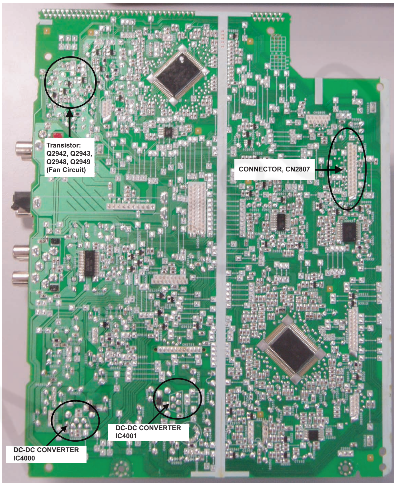
Fig. 4 Main P.C.B.
