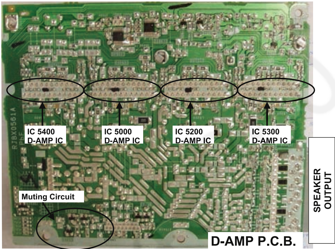
Fig. 2 D-Amp P.C.B
