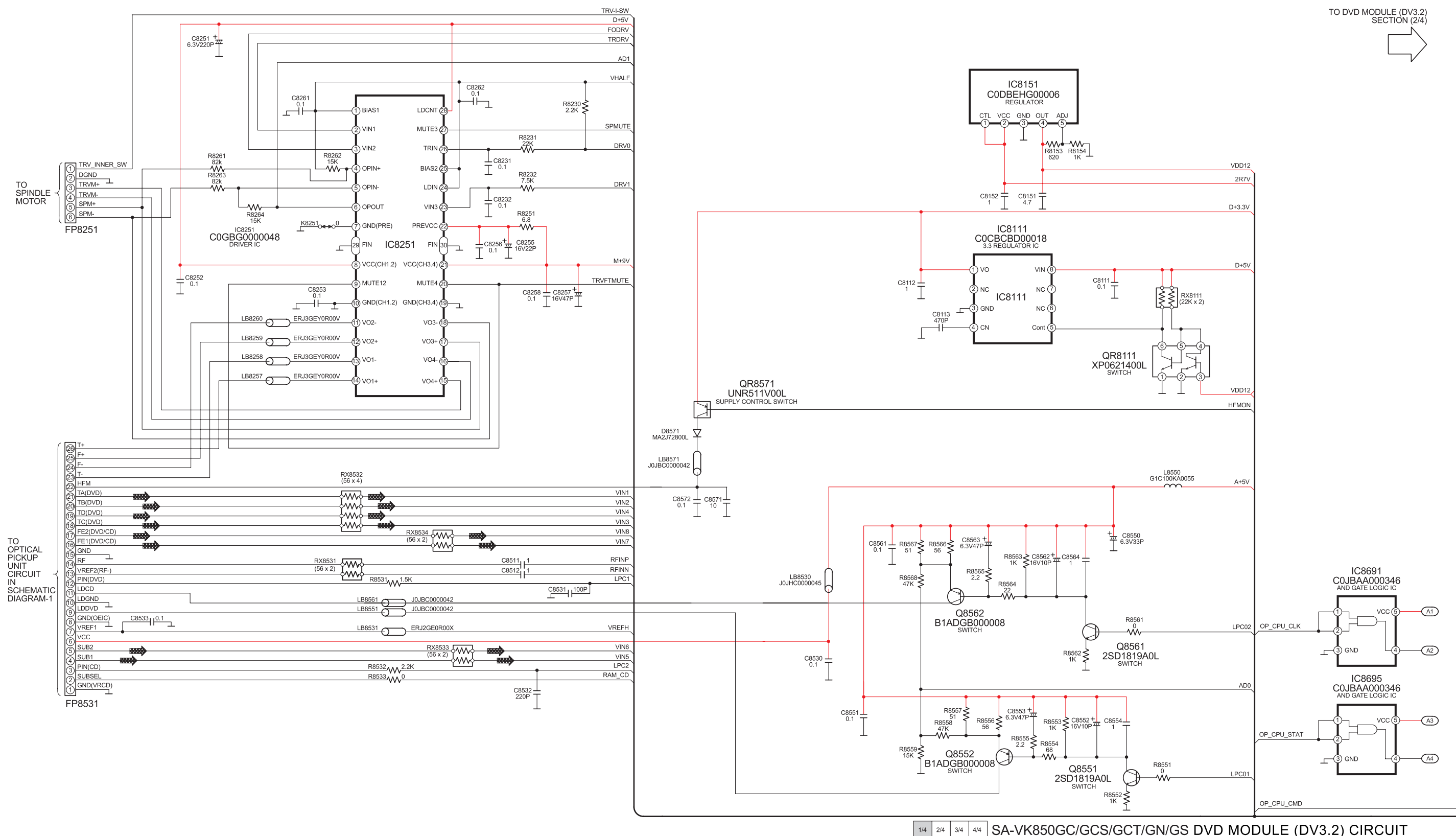
A DVD MODULE (DV3.2) CIRCUIT
