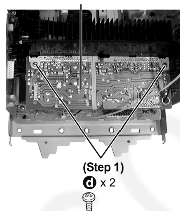
Power Amp P.C.B.
