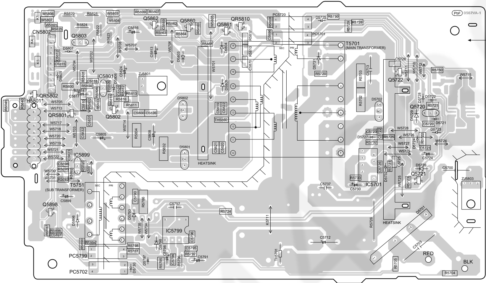
N SMPS P.C.B. (REPX0751C)
