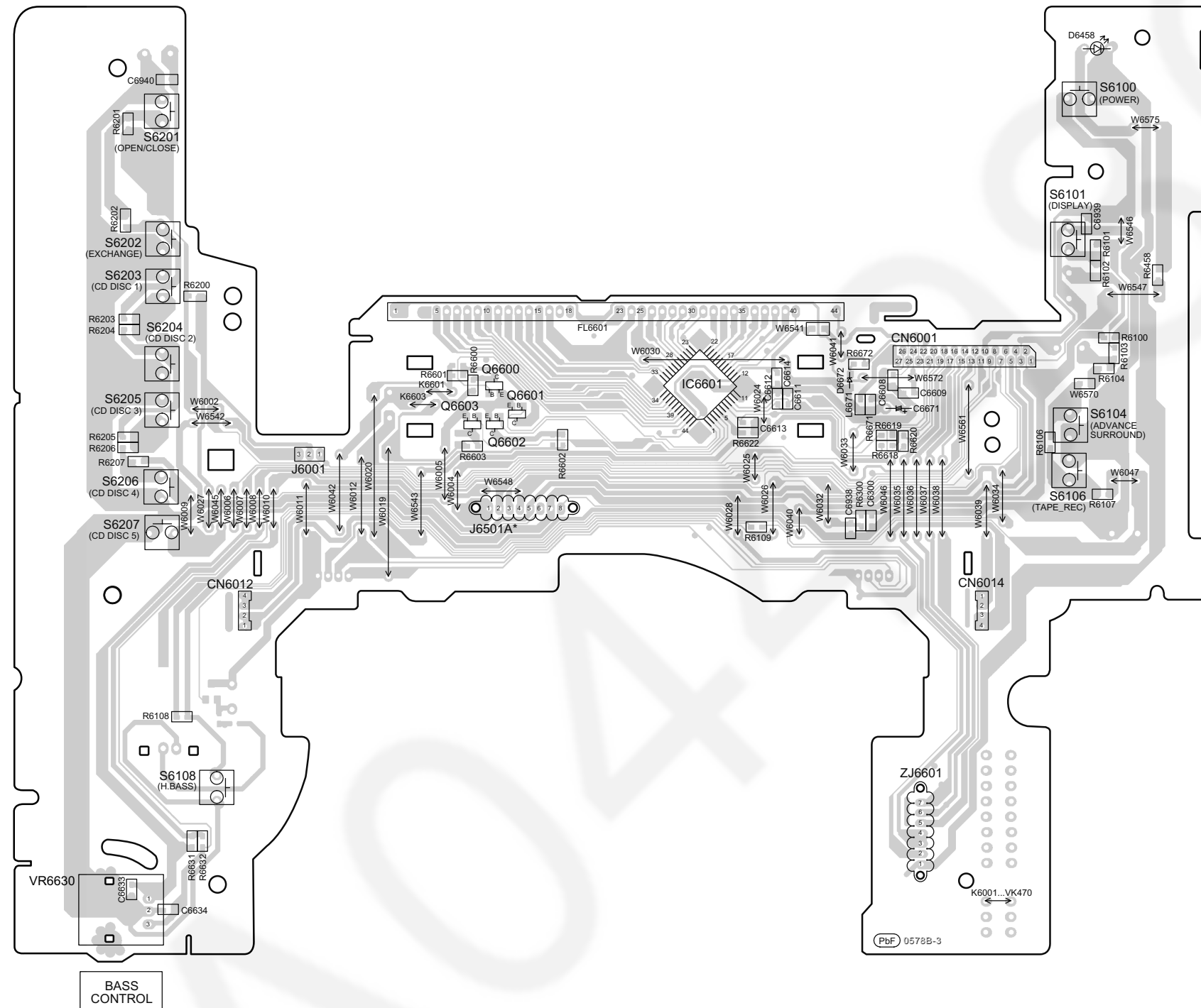
C PANEL P.C.B. (REPX0671A)
