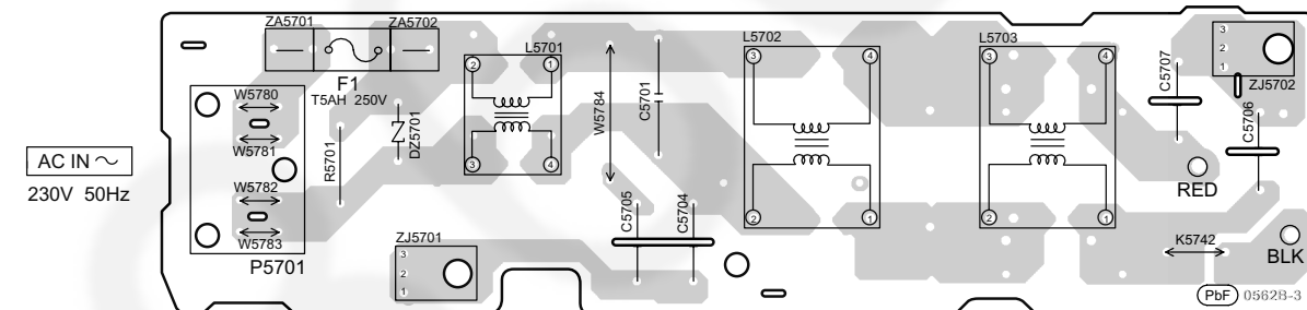
O AC INLET P.C.B. (REPX0622Y)
