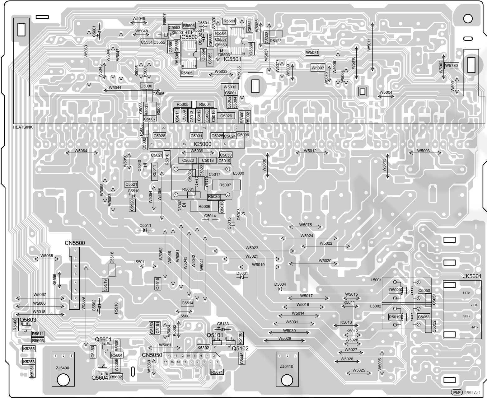
M D-AMP P.C.B. (REPX0638G)
