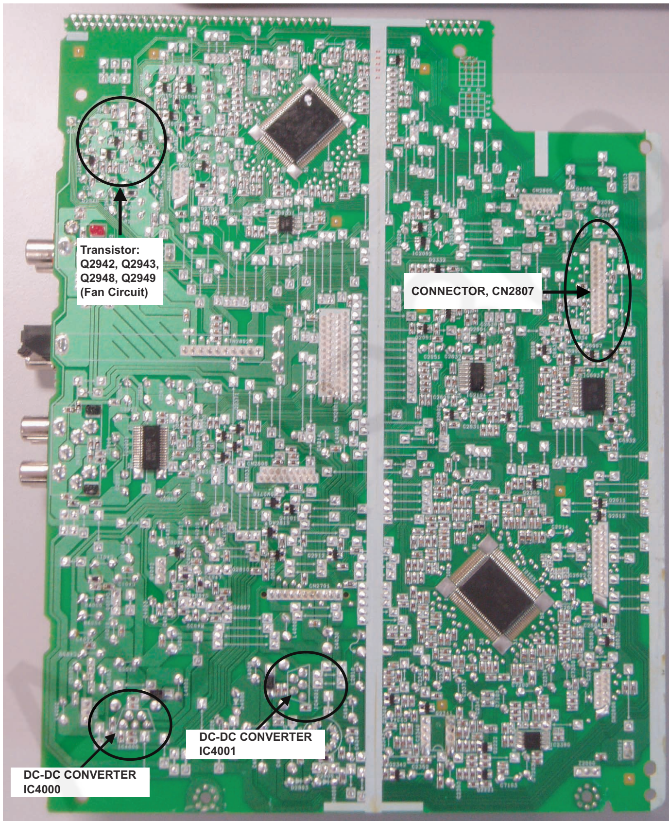
Fig. 4 Main P.C.B
