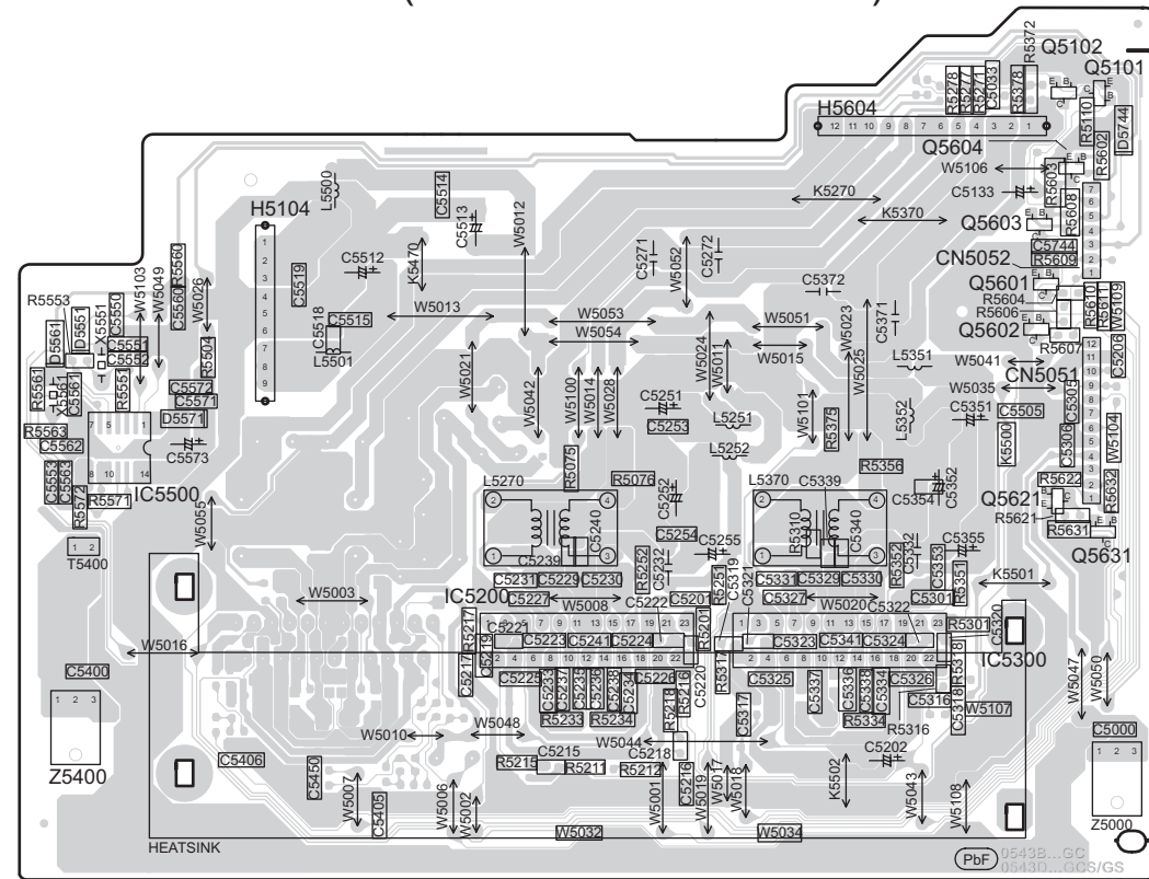
E POWER P.C.B (REPX0594B...GC) (REPX0594D...GCS/GS)
