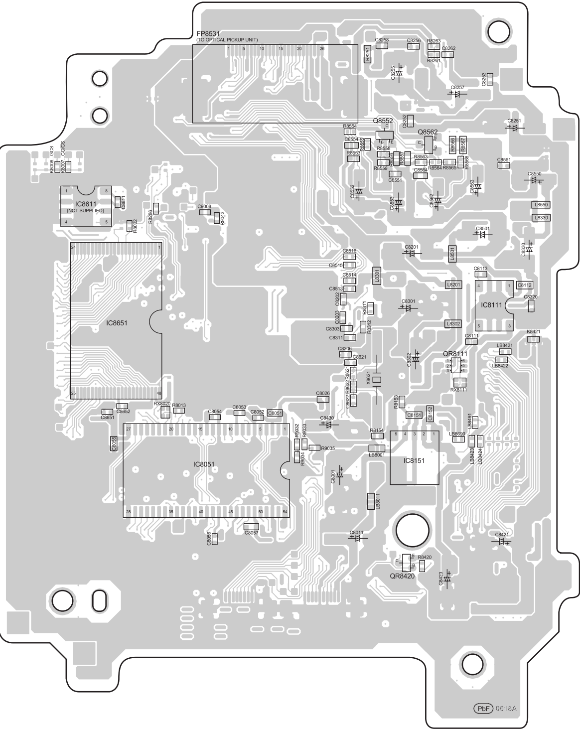
A DVD MODULE P.C.B (REPX0562C...GC/GS) (REPX0562D...GCS)
