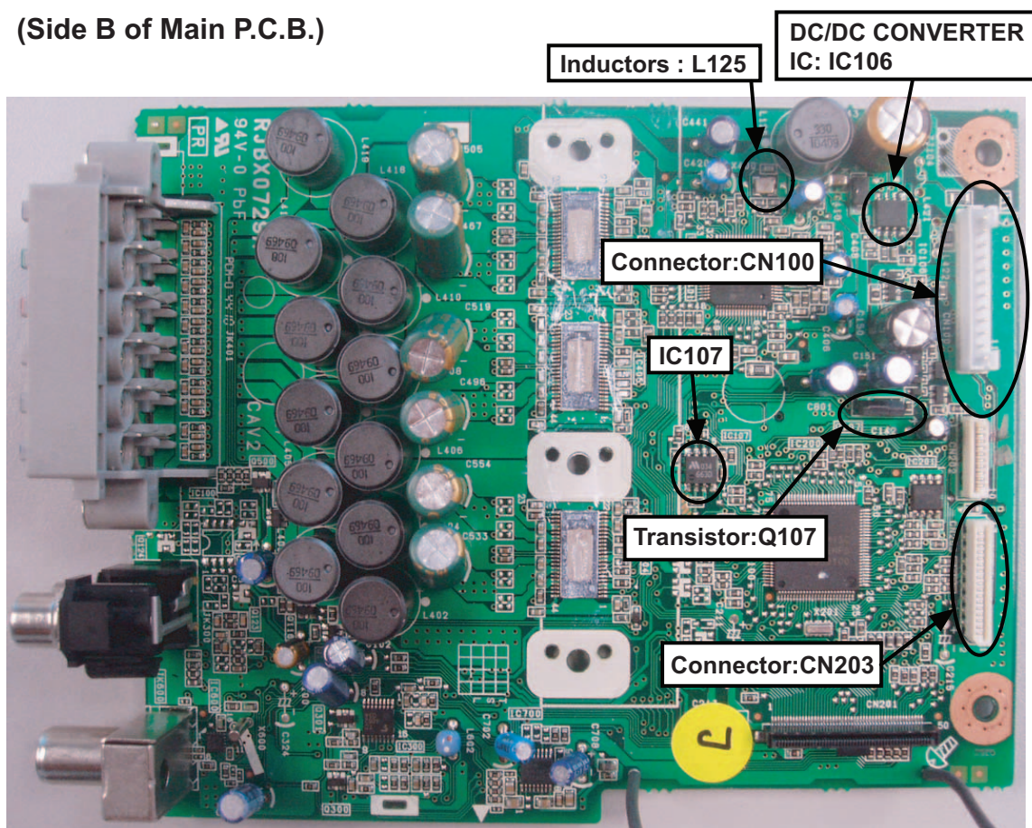
Fig. 2. Main P.C.B.
