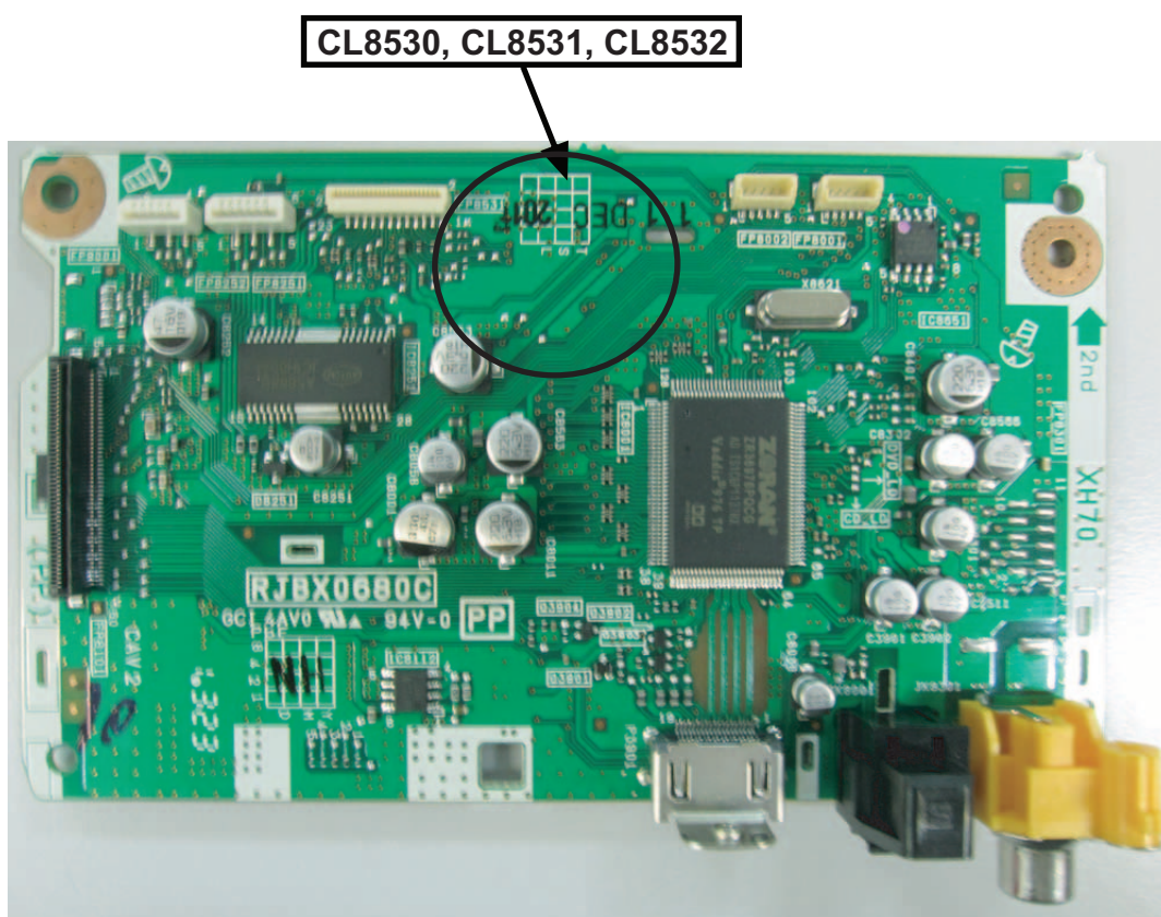
Fig. 3. Backend P.C.B.
