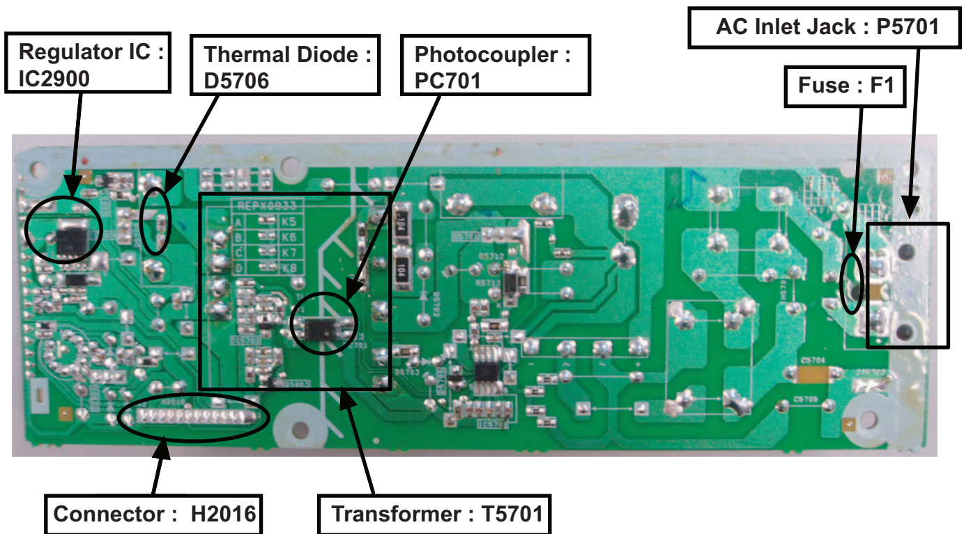
Fig. 1. SMPS P.C.B.
