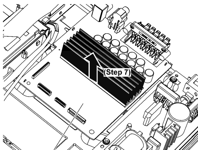
Main P.C.B.
