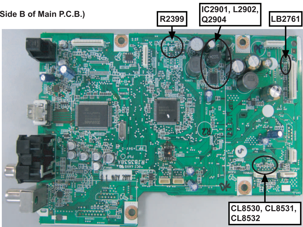
Fig. 2. Main P.C.B.
