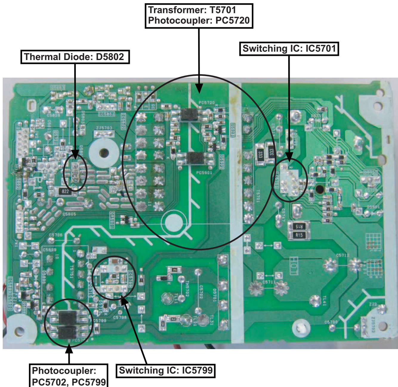
Fig. 1. SMPS P.C.B.
