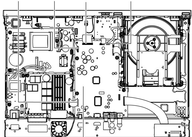
Main P.C.B.
