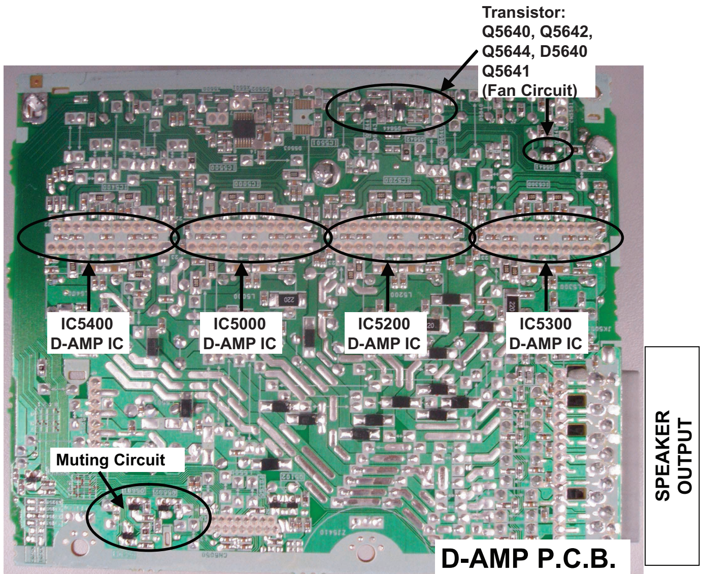
Fig. 3 D-Amp P.C.B.
