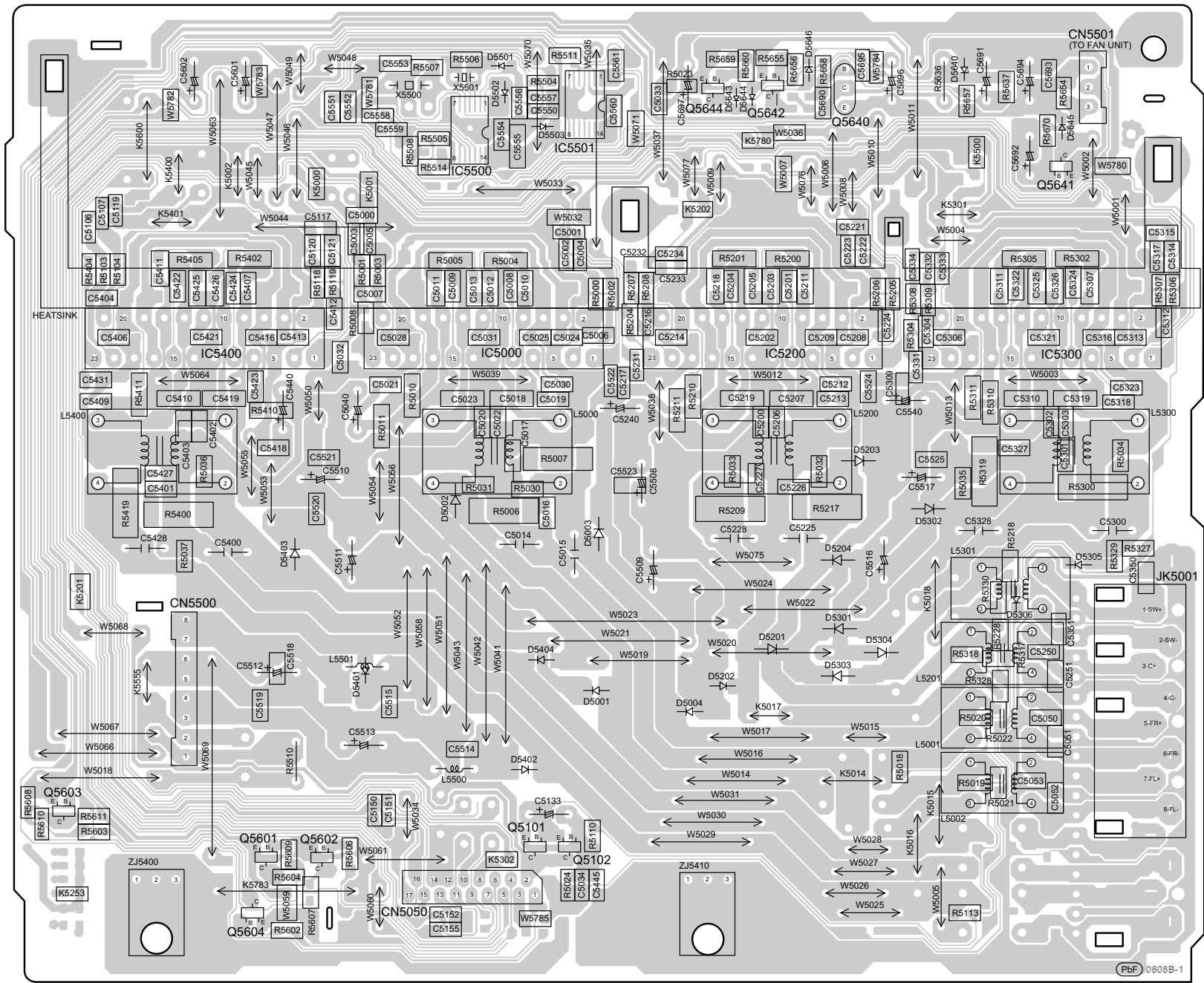
F D-AMP P.C.B. (REPX0689H)
