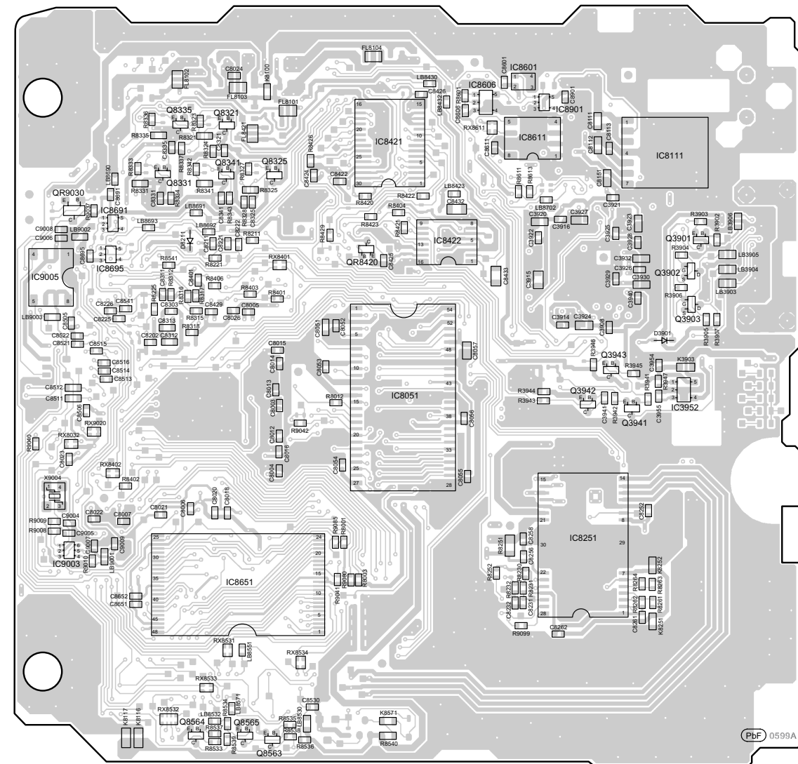
A DVD MODULE P.C.B. (RFK BX0681A-M...GC/GS) (RFK BX0681C-M...GA)
