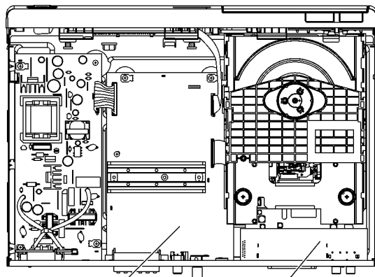
Main/D-Amp P.C.B. (Step 2)
