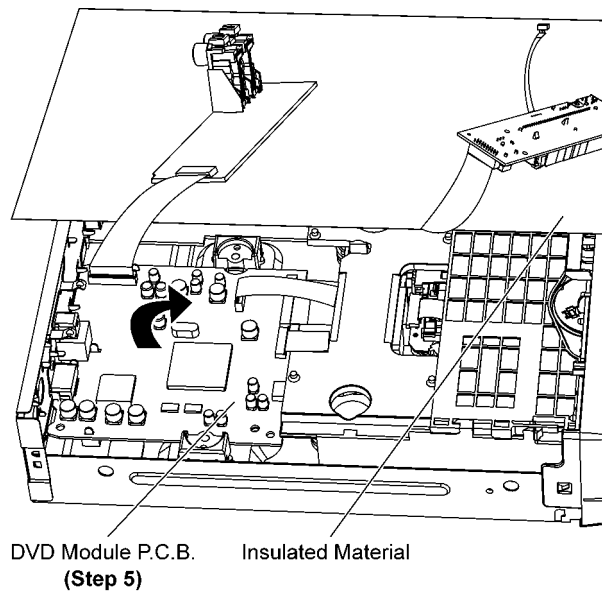
Step 5 Lift up DVD Module P.C.B..
