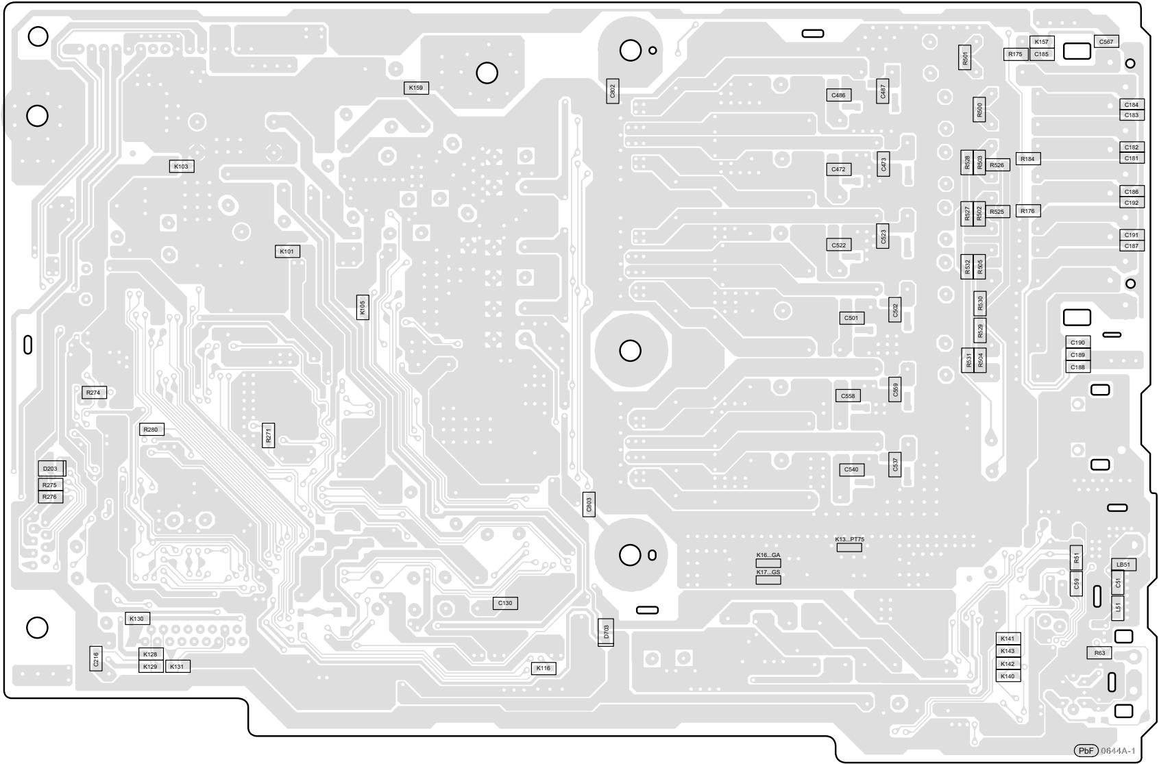
B MAIN/D-AMP P.C.B. (REPX0764K...GA) (REPX0764H...GS)
