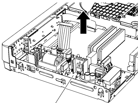
SMPS P.C.B. (Step 4)
