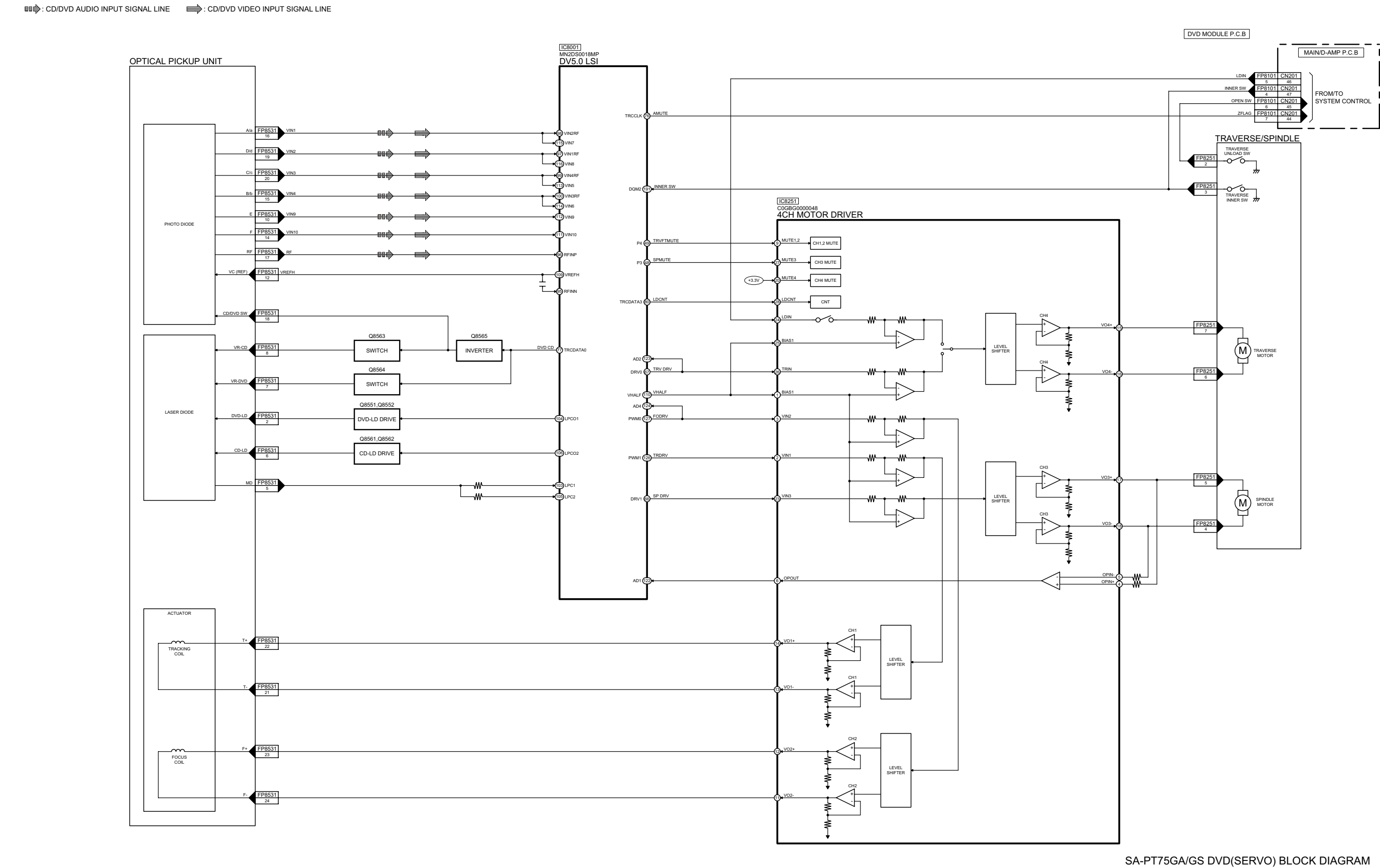
SA-PT75GA/GS DVD(SERVO) BLOCK DIAGRAM
