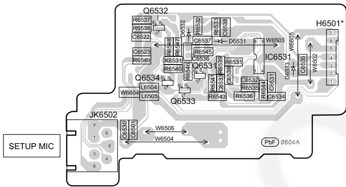
D AUTO SETUP SPEAKER P.C.B. (REPX0710A)
