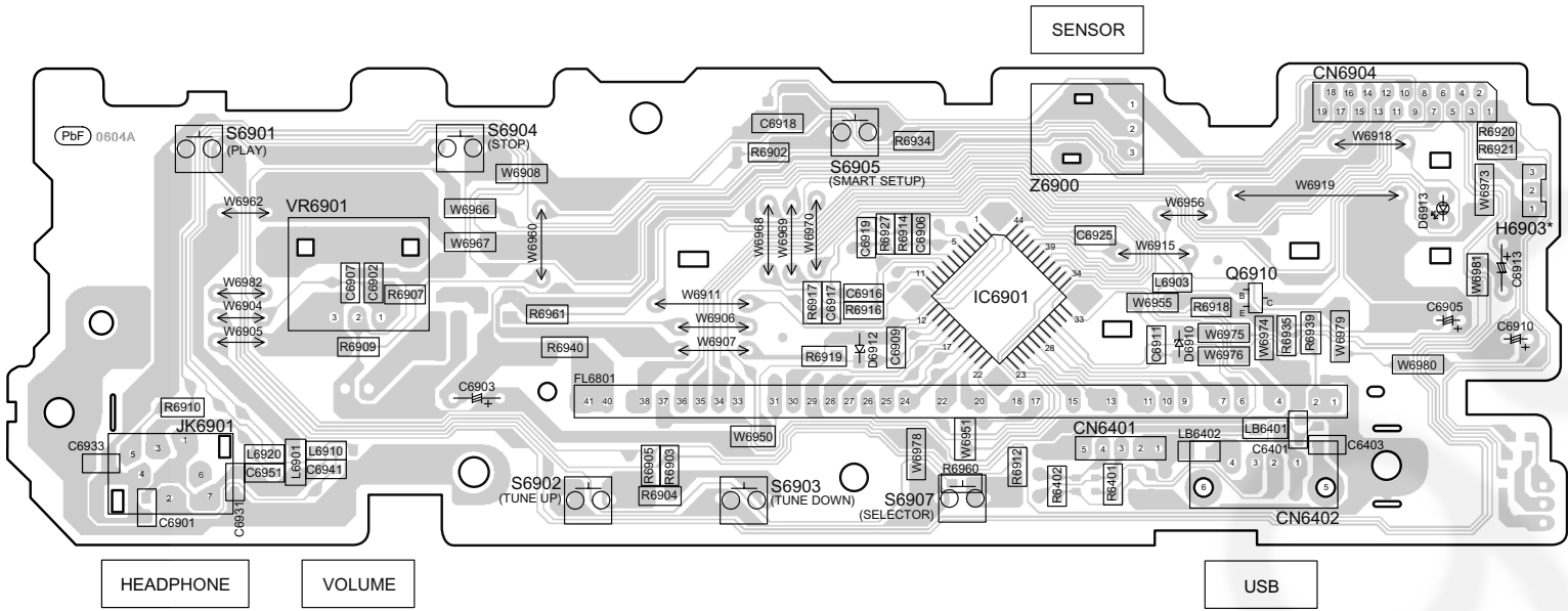
C PANEL P.C.B. (REPX0710A)
