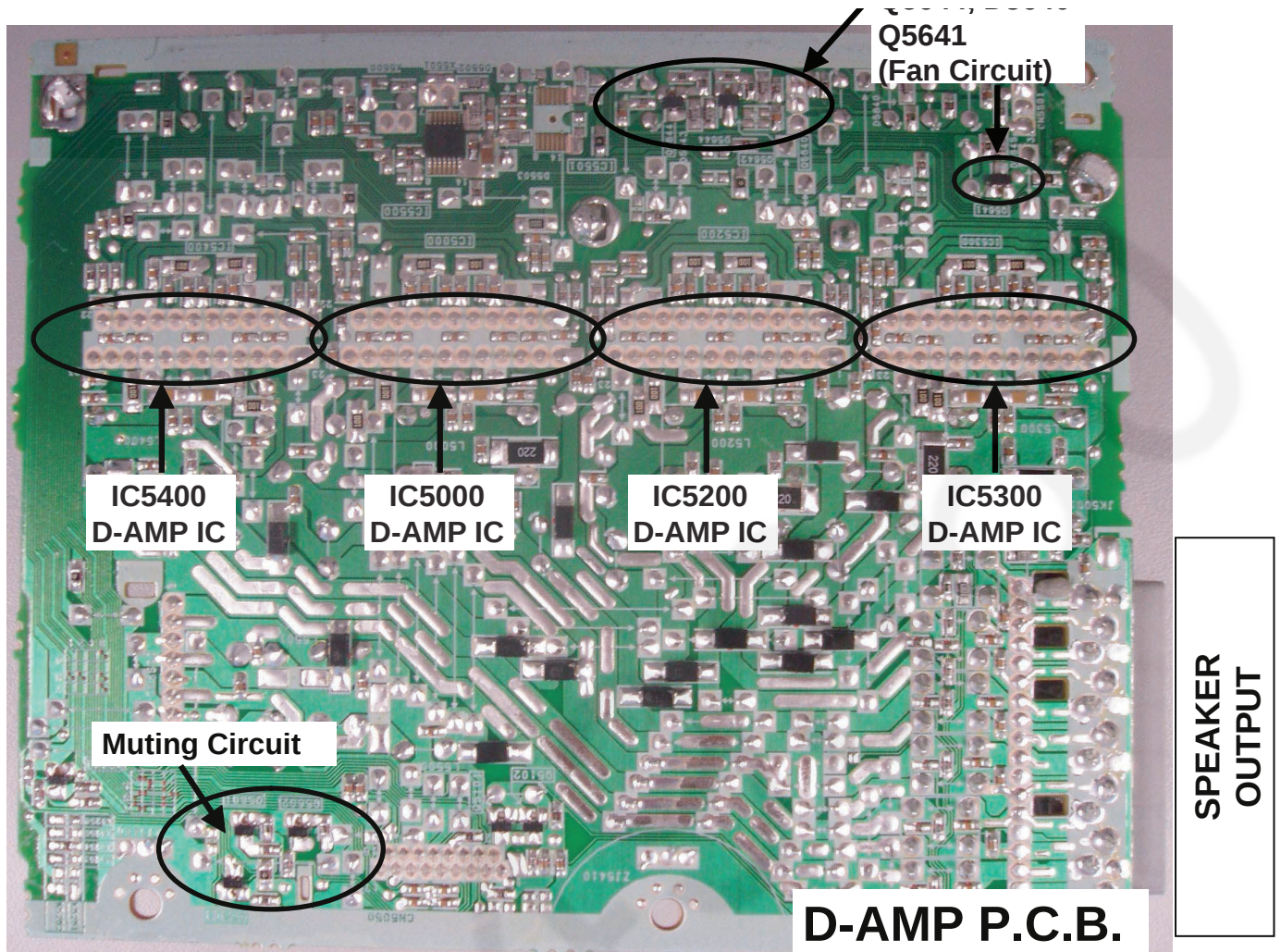
Fig. 3 D-Amp P.C.B.
