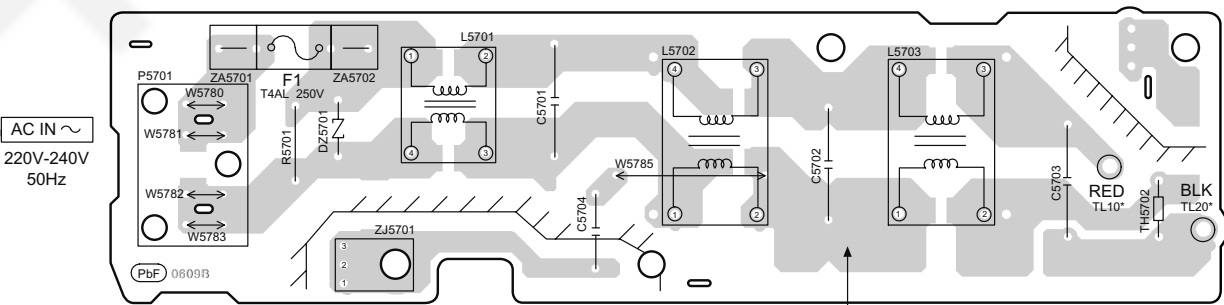
H AC INLET P.C.B. (REPX0728K)
