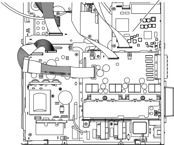
(Step 27) DVD Module P.C.B. (Side A)
