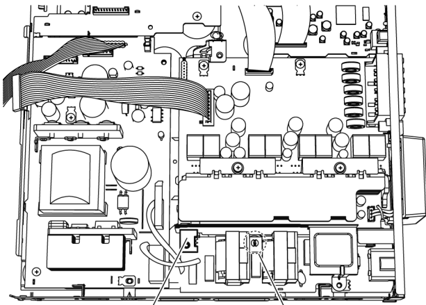
P.C.B. Bracket (Step 34)
