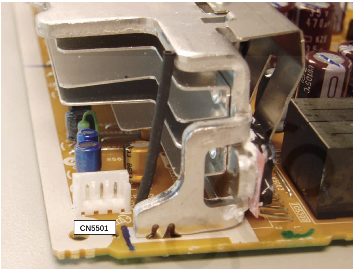
Fig. 4 Fan Connector
