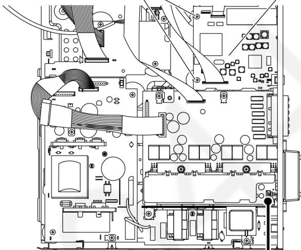
DVD Module P.C.B.
