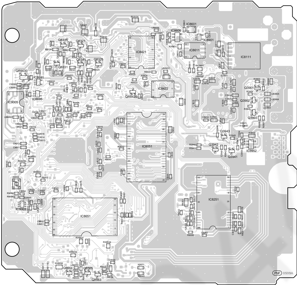
A DVD MODULE P.C.B. (RFKBB0681A-M)
