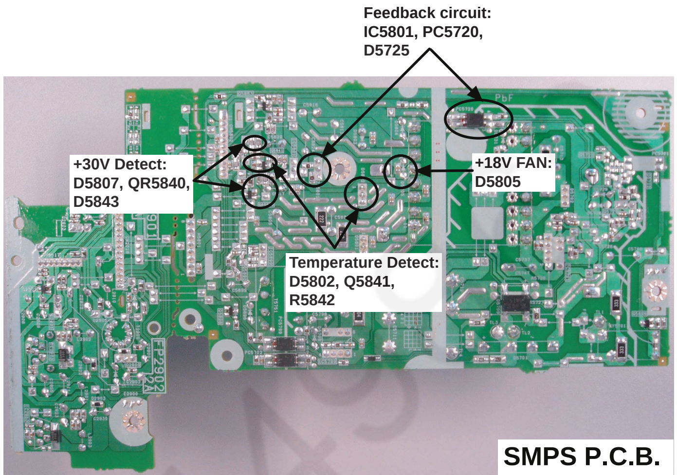
Fig.1 SMPS P.C.B.
