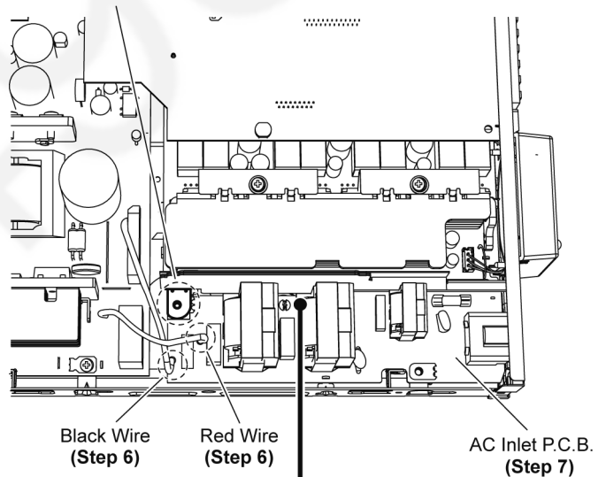
(Step 4) D-Amp P.C.B. Bracket
