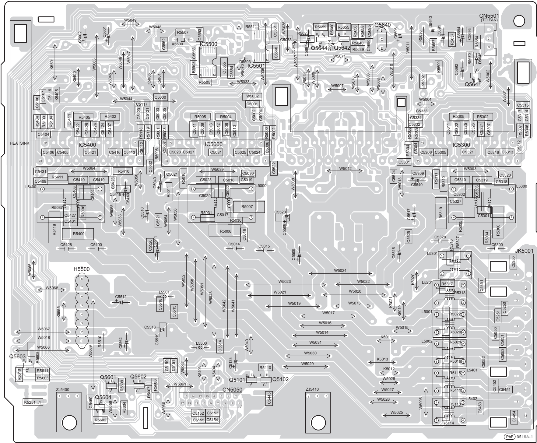
G D-AMP P.C.B. (REPX0560F)
