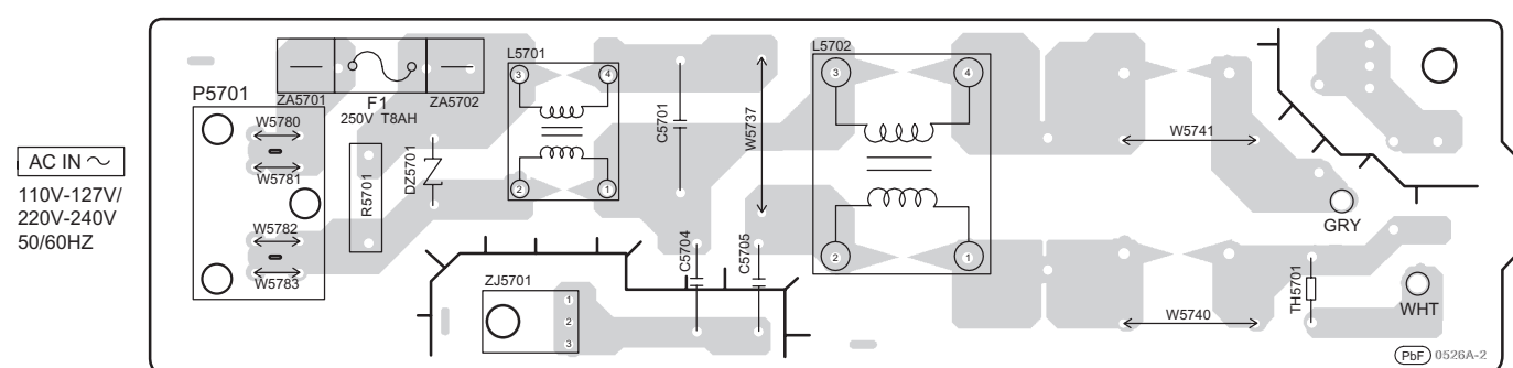
I AC-INLET P.C.B. (REPX0569B)
