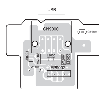
F USB P.C.B. (REPX0591H)
