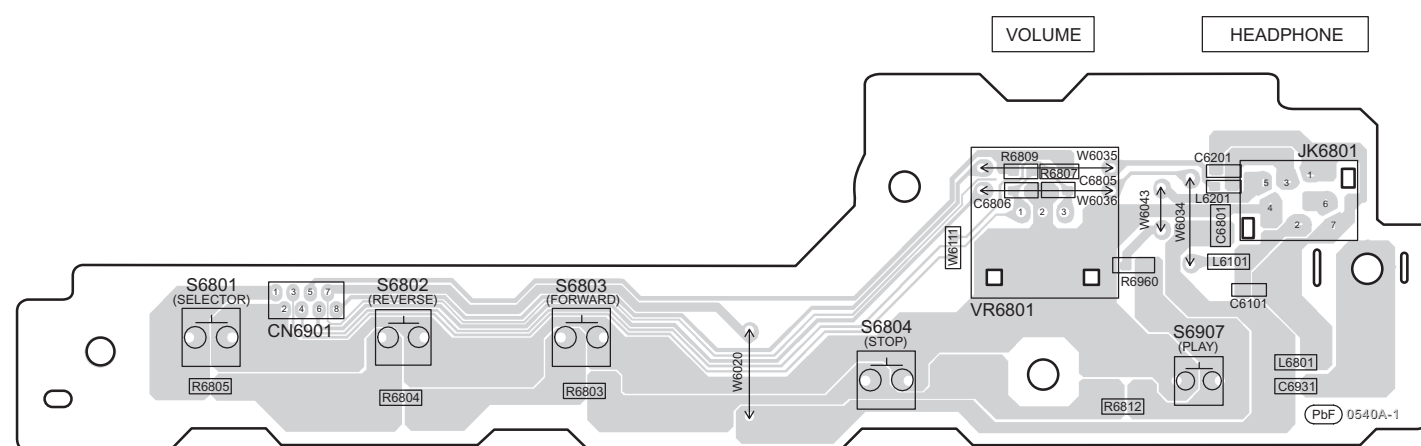
E VOLUME P.C.B. (REPX0591H)
