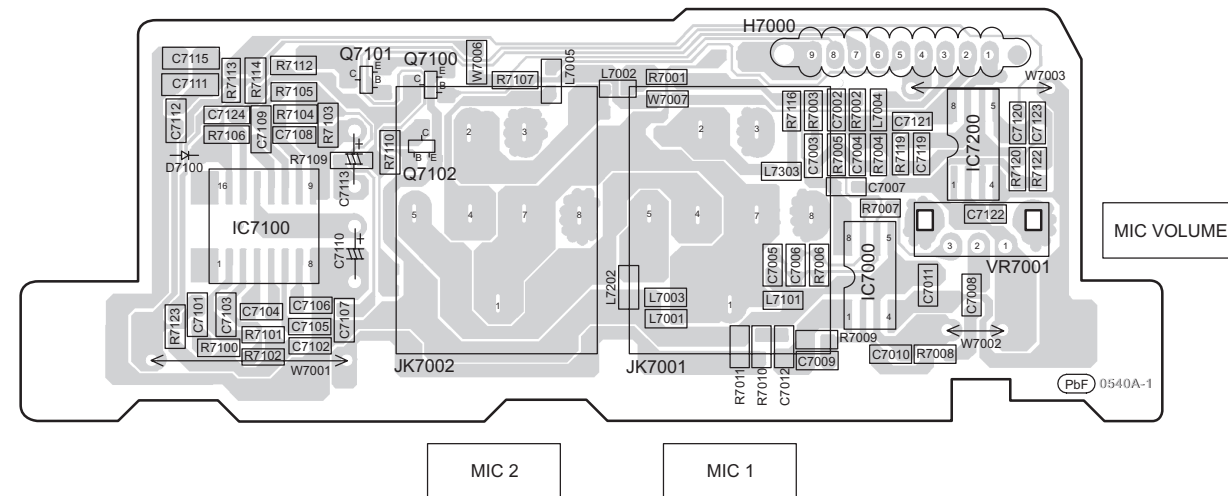
D MIC P.C.B. (REPX0591H)
