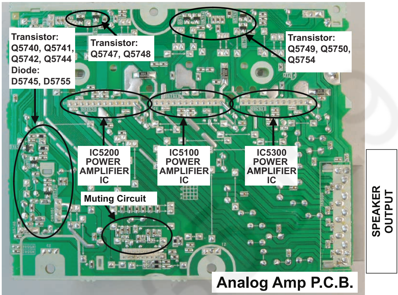
Fig. 3 Analog Amp P.C.B.
