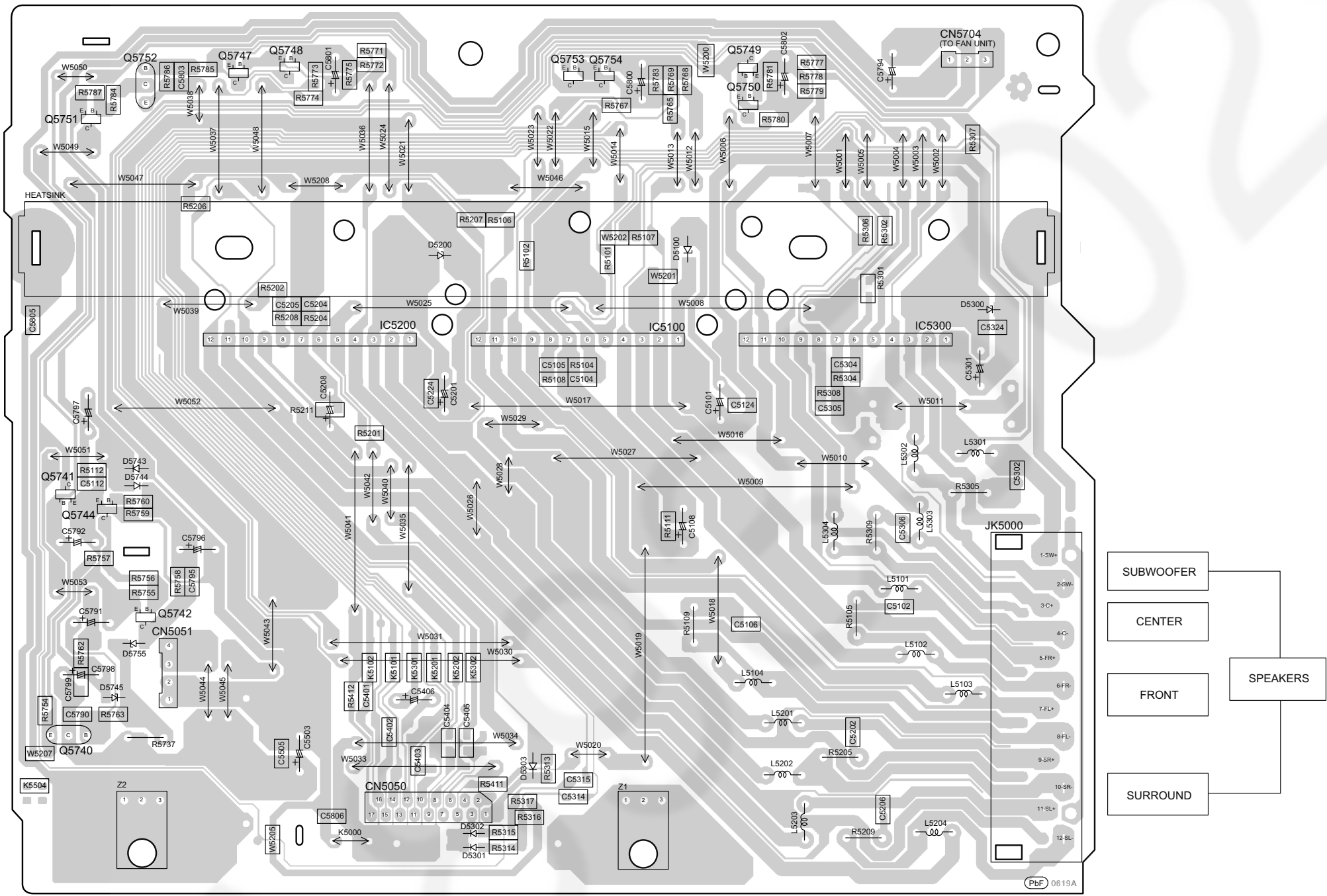
F ANALOG AMP P.C.B. (REPX0716B)
