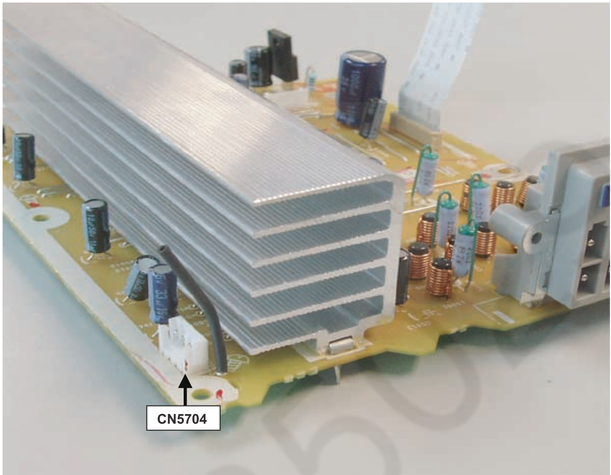
Fig. 4 Fan Connector
