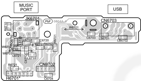
D MPORT/USB P.C.B. (REPX0710C)
