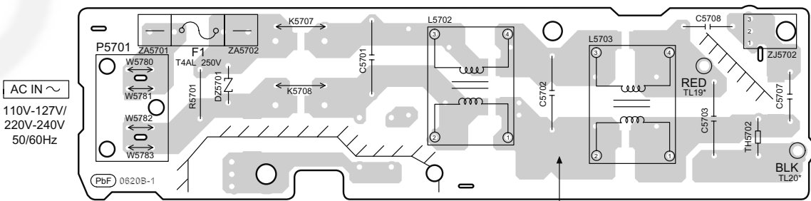
H AC INLET P.C.B. (REPX0729B)
