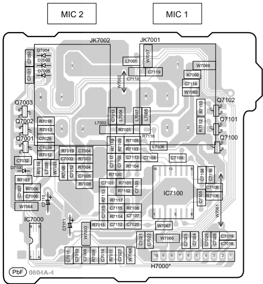
I MIC P.C.B. (REPX0710C)
