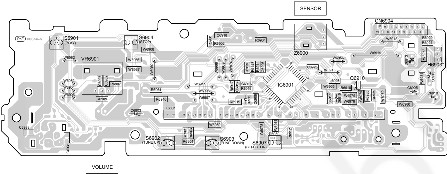
C PANEL P.C.B. (REPX0710C)
