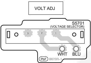
J VOLTAGE SELECTOR P.C.B. (REPX0729B)
