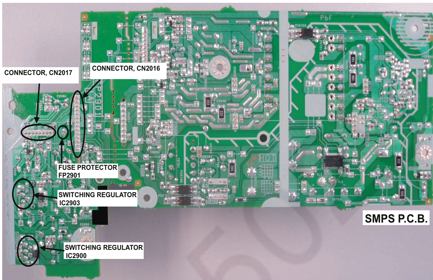
Fig. 2 SMPS P.C.B.
