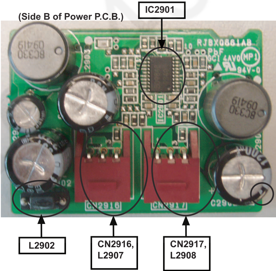
Fig 2. Power P.C.B.
