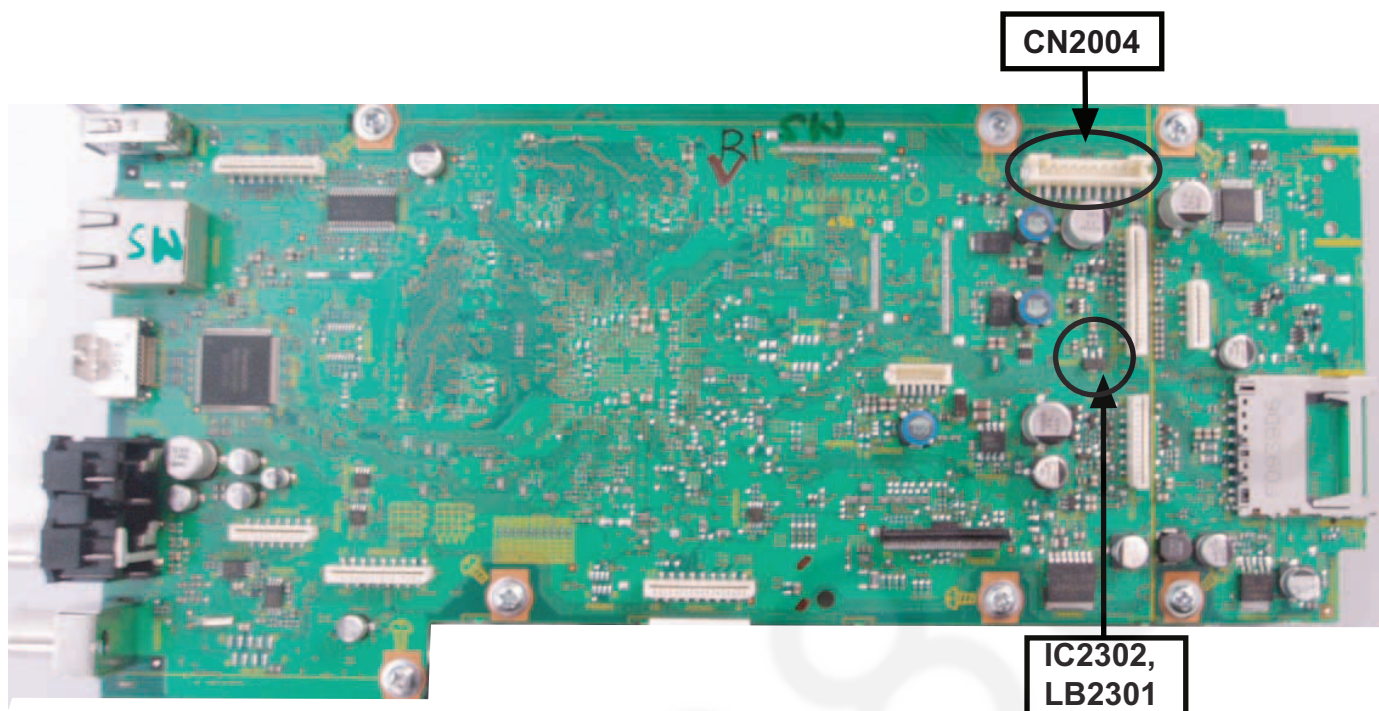
Fig 3. Main P.C.B.
