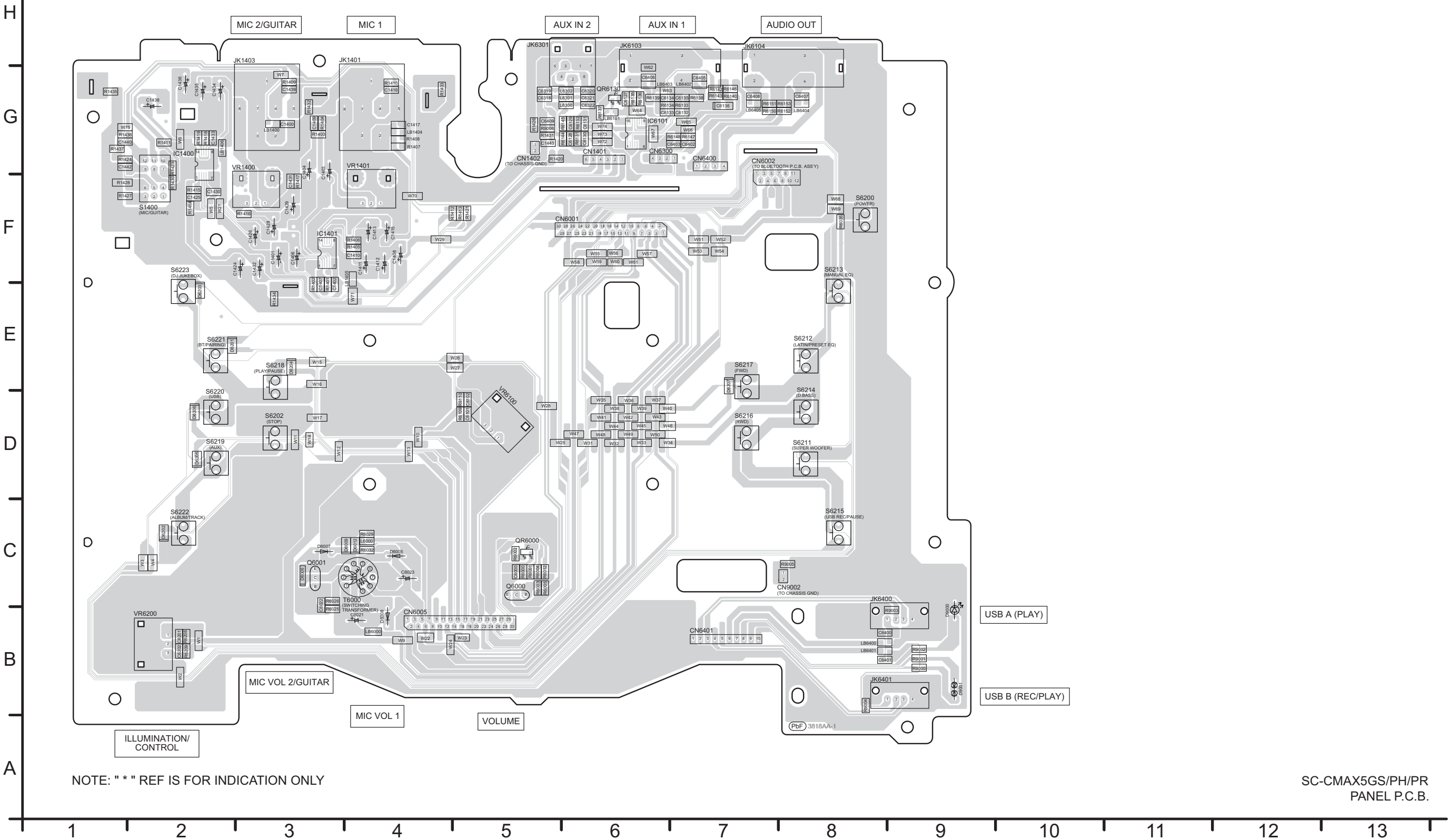
B PANEL P.C.B. (REP5106AA)
